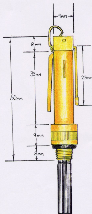
DIMENSIONS
