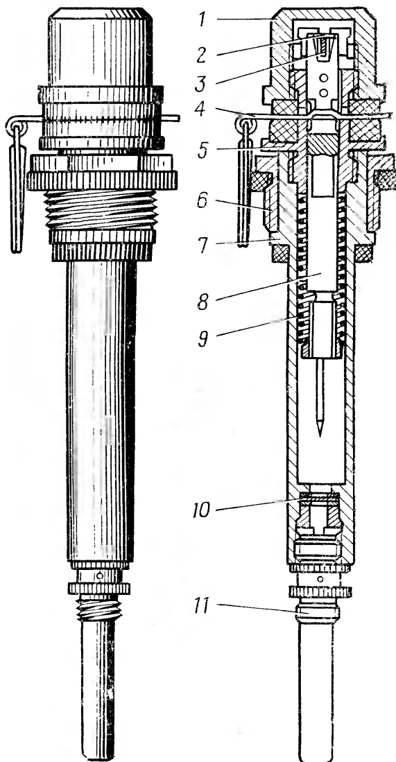
VZD-1M internal diagram
