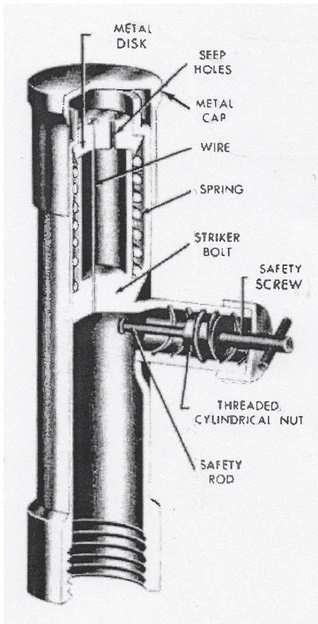
VZDKh internal diagram
