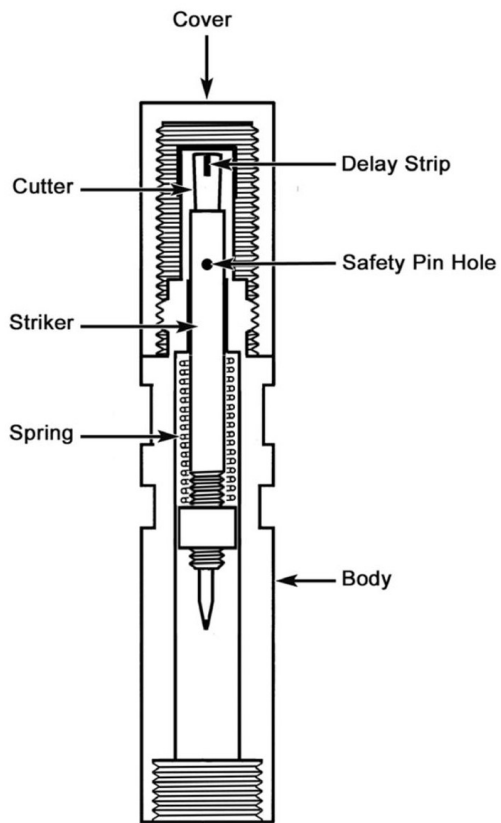
VZD-3M internal diagram
